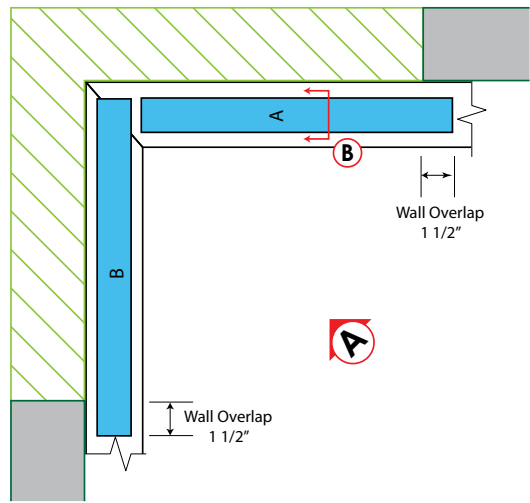
ELEVATION A
